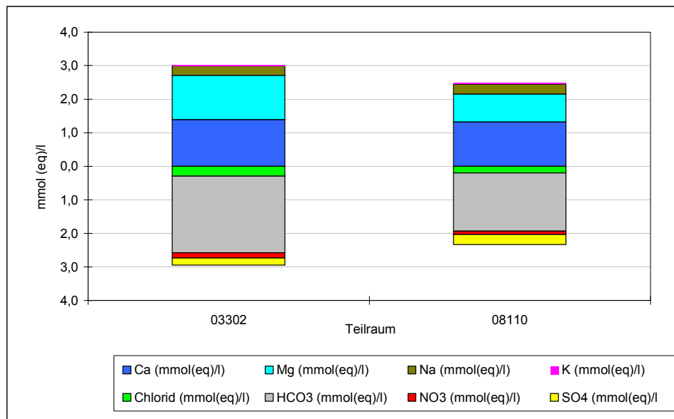
Abb. 2-4: Säulendiagramm für die hydrogeologischen Teilräume 03302 Vogelsberg und 08110 Tertiär des Westerwaldes.
