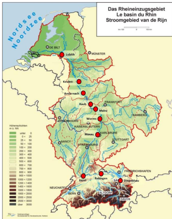
Figuur 1: Ligging van de onderzochte meetpunten aan de Rijn inclusief langjarig gemiddelde laagwaterafvoer over zeven opeenvolgende dagen (MNM7Q) (gewijzigd op basis van Bundesanstalt für Gewässerkunde - BfG)
