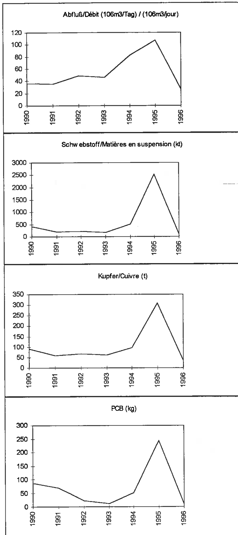
Abbildung 1: Grafische Darstellung des Zusammenhangs zwischen Abfluß, Schwebstoffjahresfracht, Jahresfracht von Kupfer und Jahresfracht von PCB bei Haringvlietsluis (siehe Tabelle 1)
