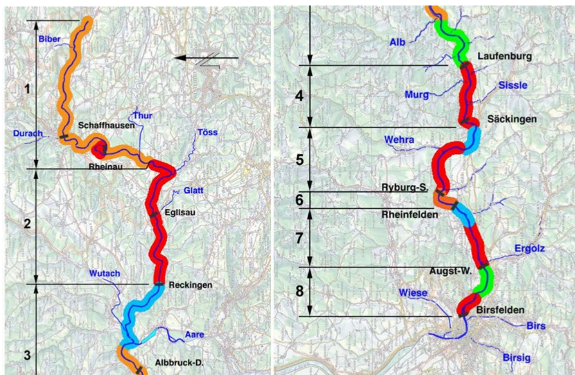
Figuur 26: Herstelpotentieel van de sedimenthuishouding in de Hoogrijn rekening houdend met bestaande waterkrachtcentrales. Schaal 1 : 400'000; ■ Stuw; Herstelpotentieel ■ zeer groot, ■ groot, ■ gemiddeld, ■ klein / verwaarloosbaar
