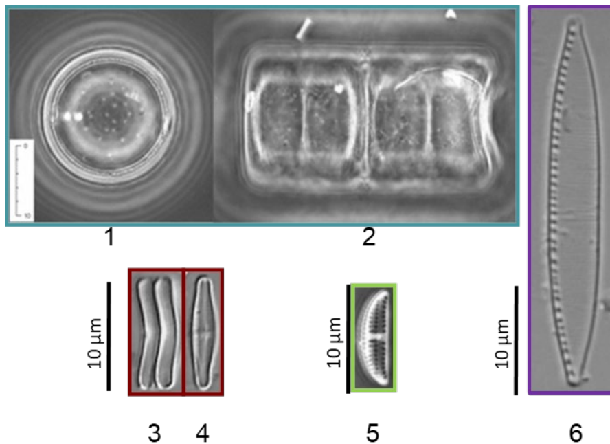
Figuur 40: Foto's van de vier meest differentiërende soorten benthische kiezelalgen (diatomeeën) op de verschillende Rijntrajecten 1-2: Melosira varians valvazijde (1) en pleurazijde (2); 3-4: Achnantheidium minutissimum sensu lato pleurazijde (3) en valvazijde (4); 5: Amphora pediculus ; 6: Nitzschia palea . Foto's: D. Heudre.
