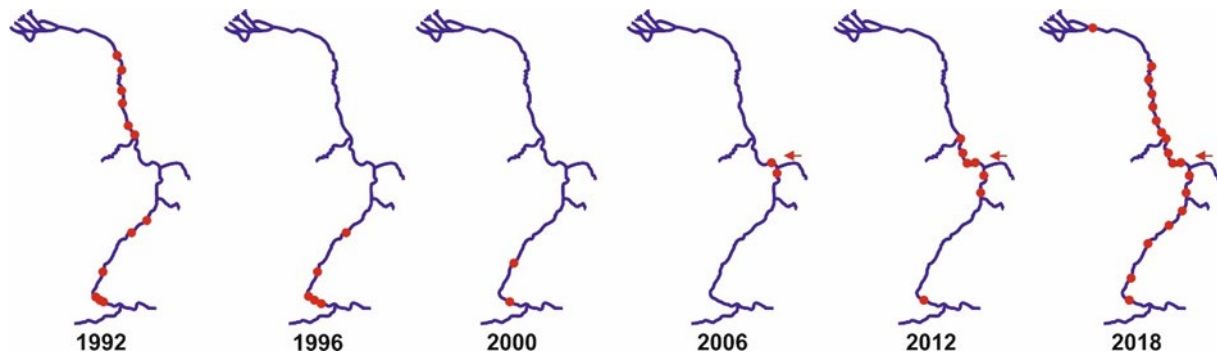
Figuur 42: Verspreiding van de zoetwaterneriet Theodoxus fluviatilis in de bevaarbare Rijn (Westermann et al. 2007, aangevuld), er is geen rekening gehouden met het voorkomen in zijrivieren
