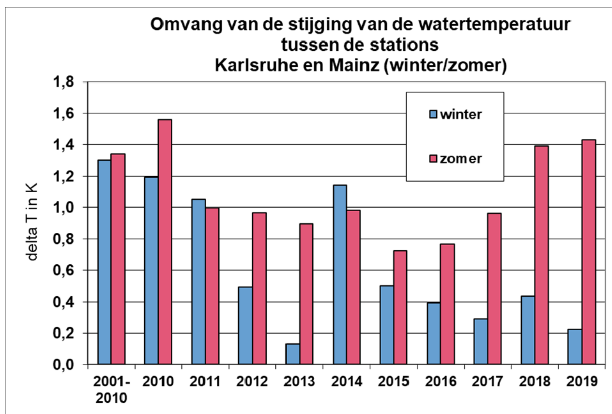
Figuur 10: Omvang van de stijging van de watertemperatuur (winter = jan-mrt, okt-dec; zomer = apr-sept), uitgedrukt in Kelvin, tussen Karlsruhe en Mainz (figuur: SGG Rijn)
