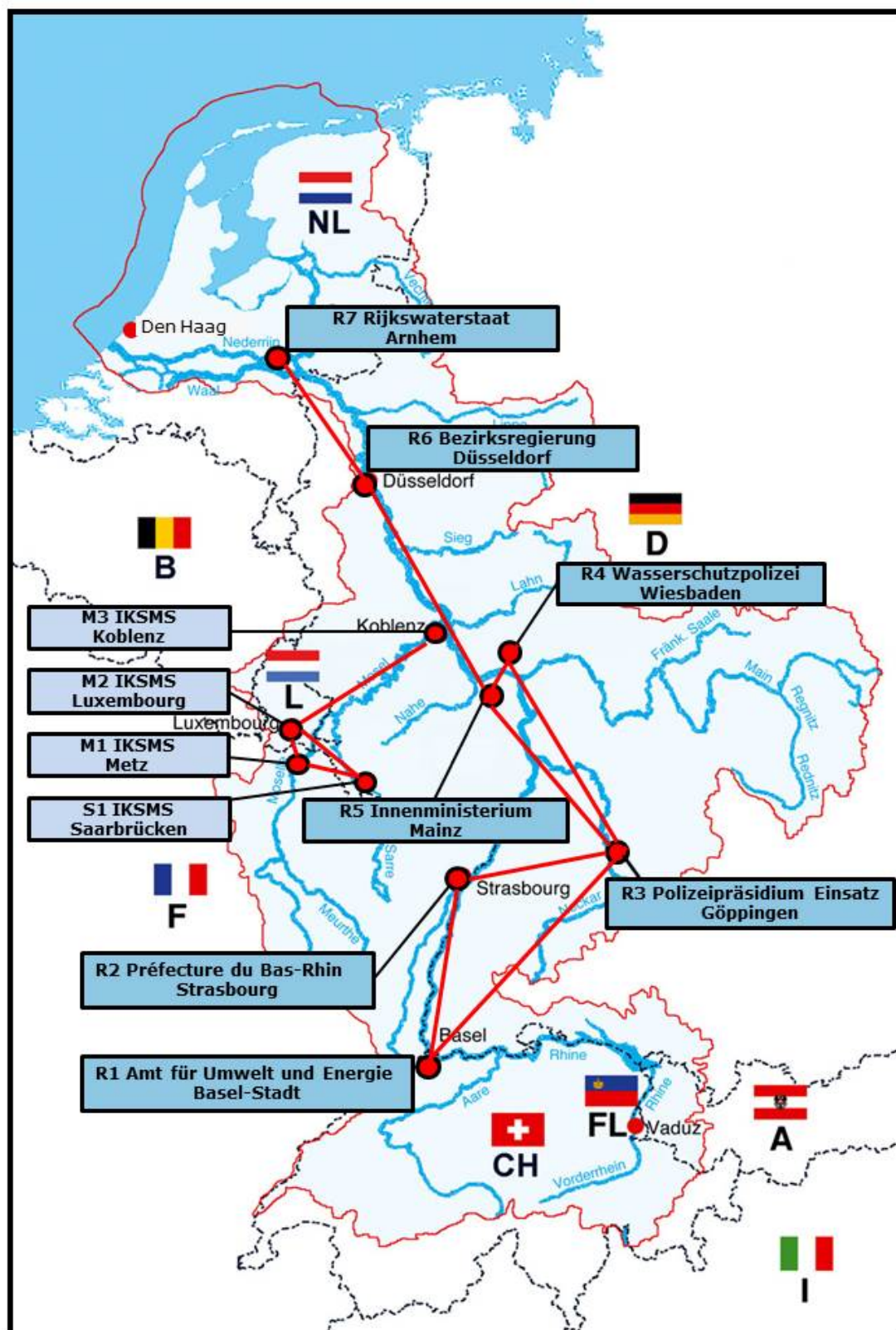
Figure 45 : centres Principaux Internationaux d'Avertissement - mise à jour : 2014
