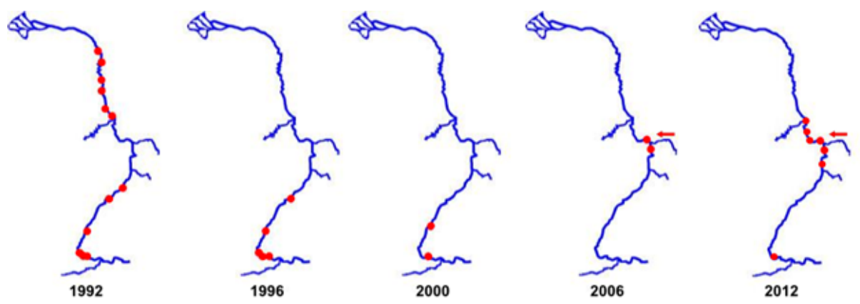
Figure 16 : propagation de la nérîte des rivières Theodoxus fluviatilis dans le Rhin navigable (Westermann et al. 2007, complété), les affluents ne sont pas pris en compte.
