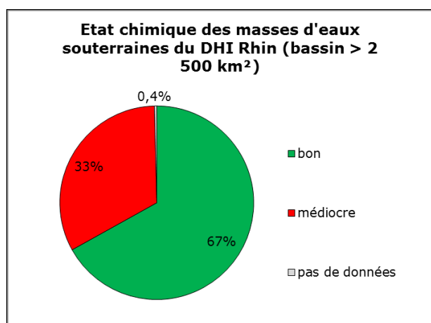
Figure 27 : état chimique actuel des masses d'eaux souterraines dans le DHI Rhin (bassin > 2 500 km²). Mise à jour des données : décembre 2015 ; données sans la Suisse, voir texte de la figure 10
