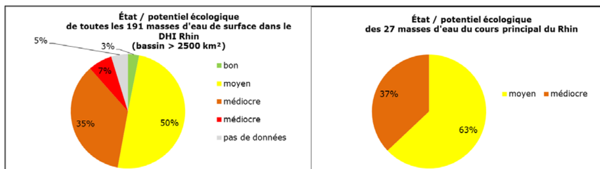
Figure 10 : état/potentiel écologique de toutes les masses d'eau de surface dans le DHI Rhin (bassin > 2 500 km 2 , à gauche) et des masses d'eau sur le cours principal du Rhin (à droite) sur la base du nombre de masses d'eau (mise à jour : décembre 2015). Données sans la Suisse, voir ci-dessous
