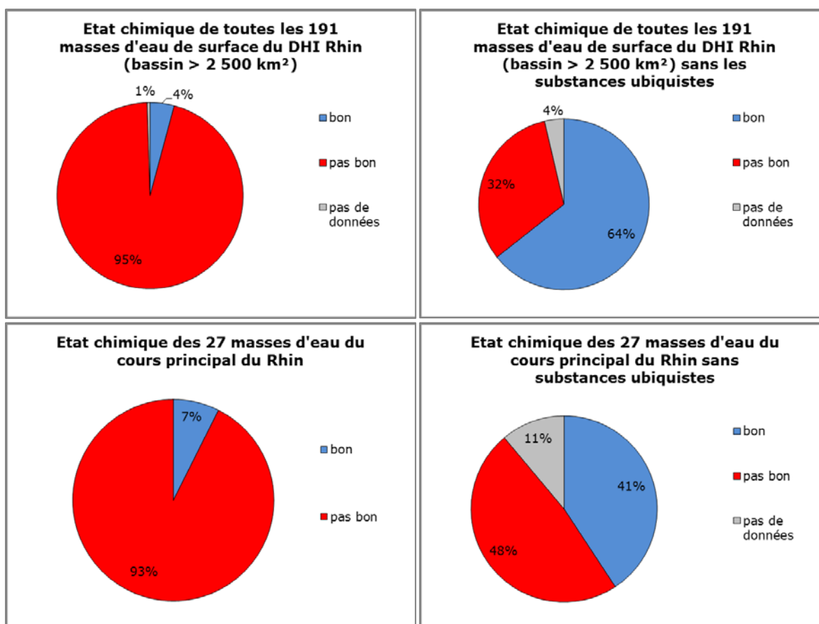
Figure 25 : état chimique actuel (résultats d'évaluation 2012/2013) de toutes les masses d'eau de surface dans le DHI Rhin (bassin > 2 500 km 2 , en haut) et des masses d'eau du cours principal du Rhin (en bas) avec (à gauche) et sans (à droite) substances ubiquistes. Evaluation nationale actuelle conforme à la directive 2013/39/UE. Mise à jour des données : décembre 2015 ; données sans la Suisse, voir texte de la figure 10
