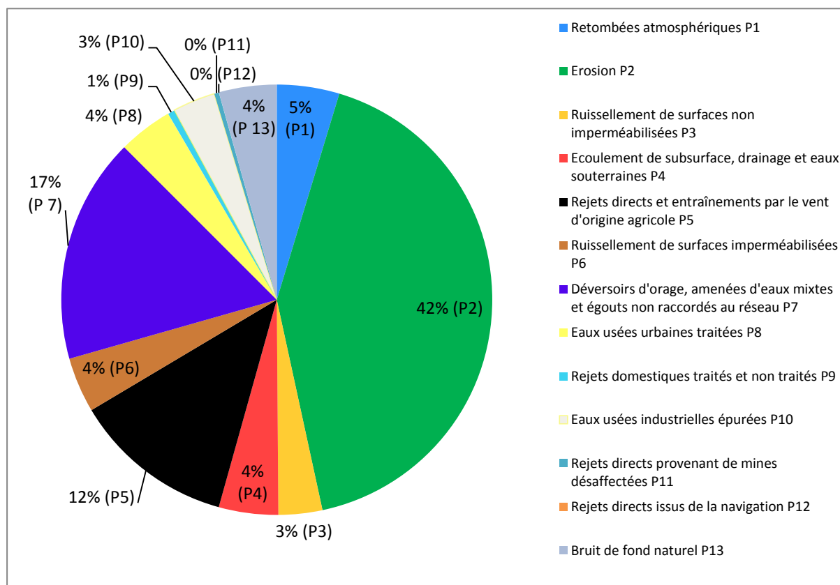
Figure 5 : répartition des apports de plomb sur les voies d'apport en 2010 (apport total de 150 t) 15 .
