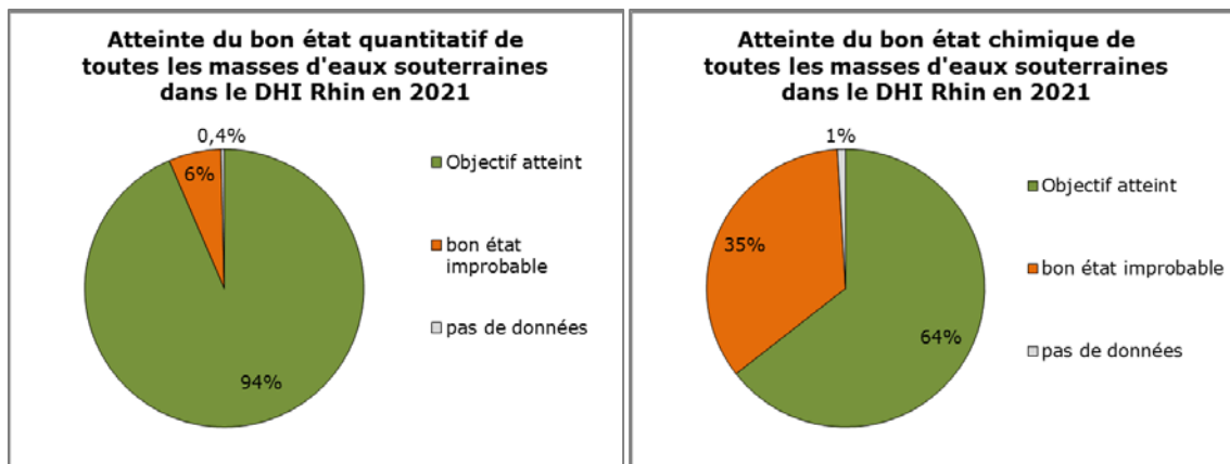
Figure 31 : atteinte de l'objectif quantitatif (à gauche) et de l'état chimique (à droite) en 2021 dans toutes les masses d'eaux souterraines du DHI Rhin. Mise à jour des données : décembre 2015 ; données sans la Suisse, voir texte de la figure 10
