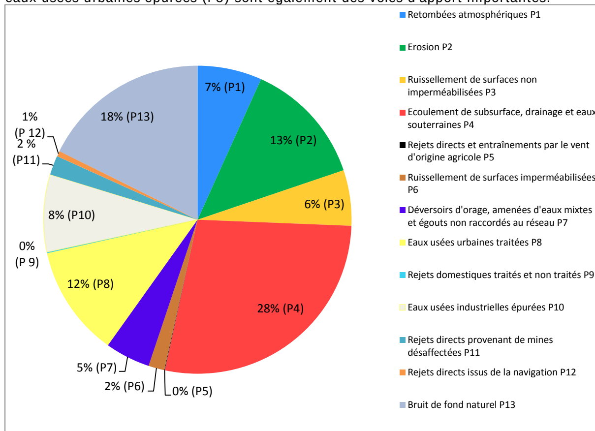
Figure 6 : répartition des apports de cadmium sur les voies d'apport en 2010 (apport total de 3,96 t) 15 .
