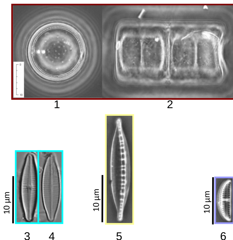
Figure 15 : photos de 4 espèces de diatomées structurantes dans les différents tronçons du Rhin 1-2: Melosira varians vue de dessus (1) et de côté (2) ; 3-4: Achnanthes pyrenaicum , 5: Nitzschia dissipata ; 6: Amphora pediculus ; Photos D. Heudre)
