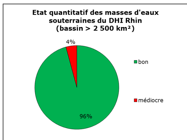
Figure 26 : état quantitatif actuel des masses d'eaux souterraines dans le DHI Rhin (bassin > 2 500 km²). Mise à jour des données : décembre 2015 ; données sans la Suisse, voir texte de la figure 10
