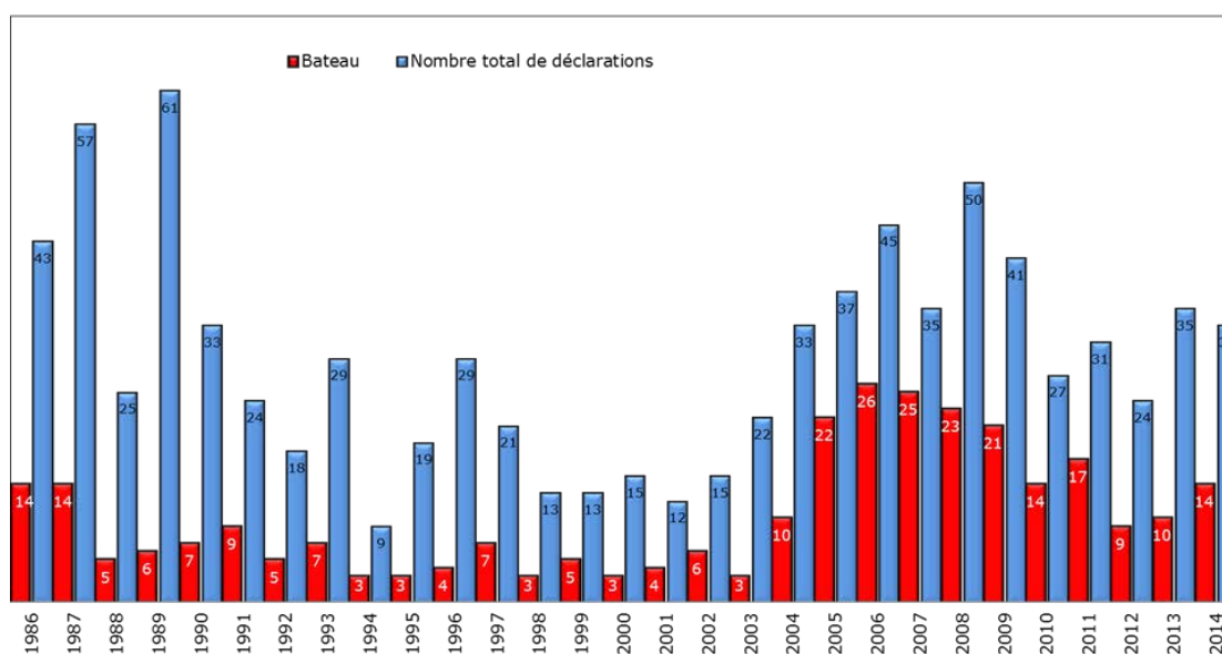
Figure 44 : évolution du nombre de déclarations imputables à des bateaux entre 1986 et 2014 par rapport au total de déclarations.
